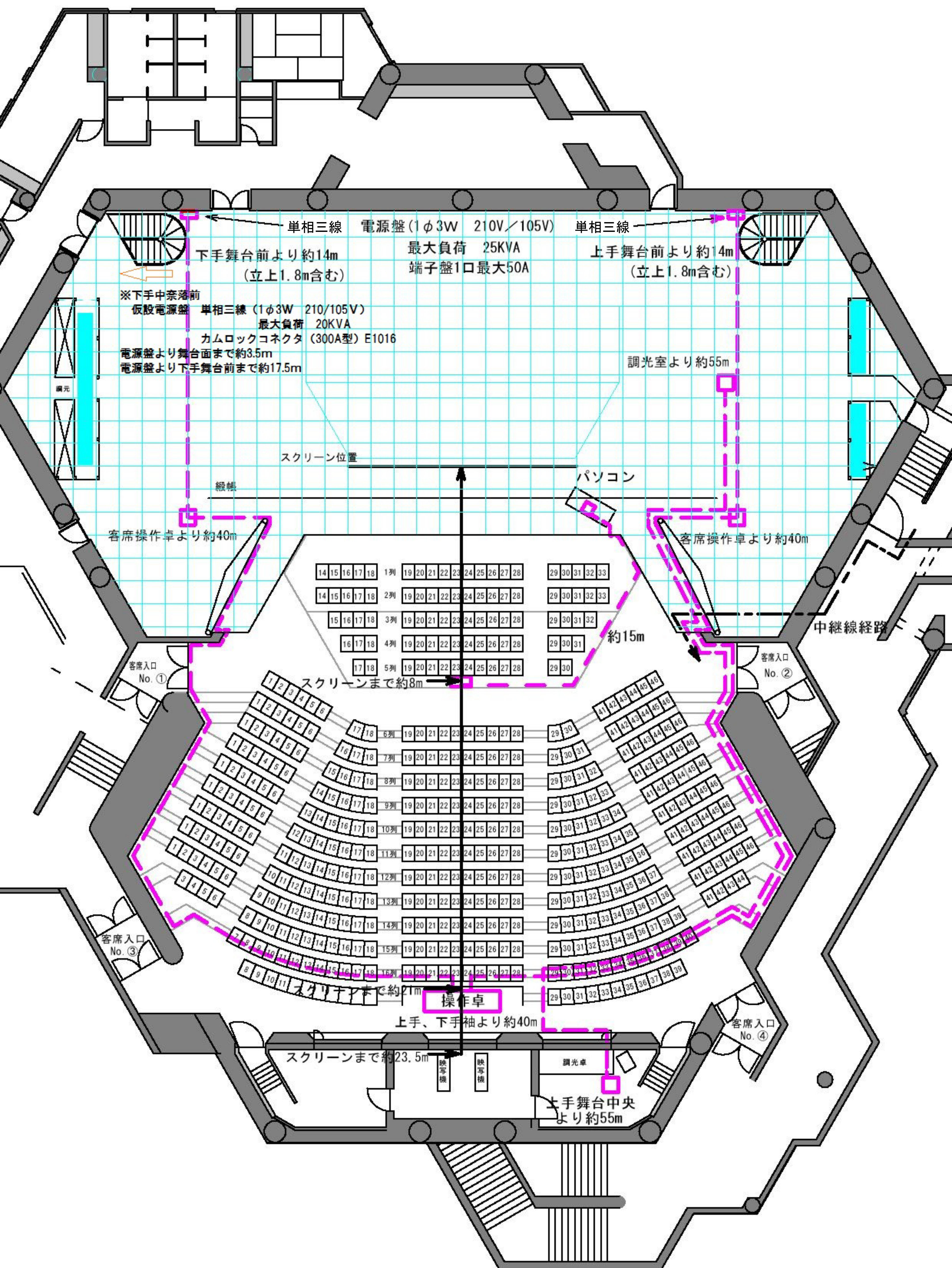
ホール平面図（ケーブル距離）
