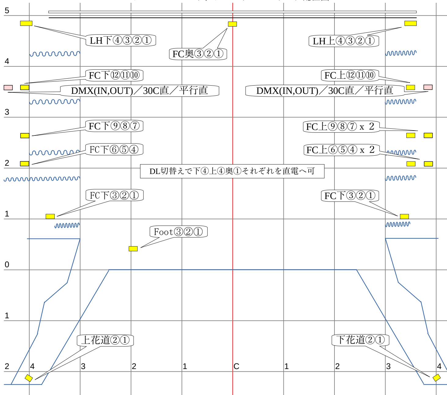
ステージコンセント、フロント・シーリング配置図
