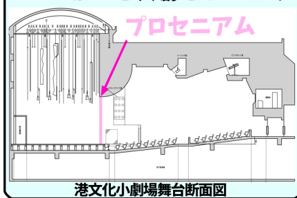
港文化小劇場舞台断面図
