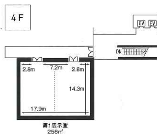
名古屋市民ギャラリー矢田 展示室平面図
